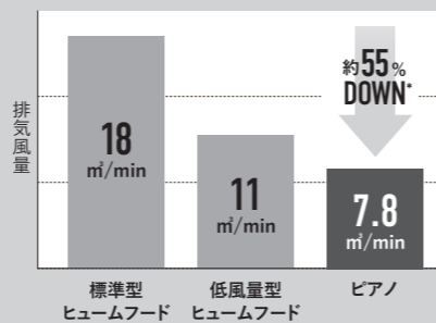
排気装置タイプ別の排気風量比較
